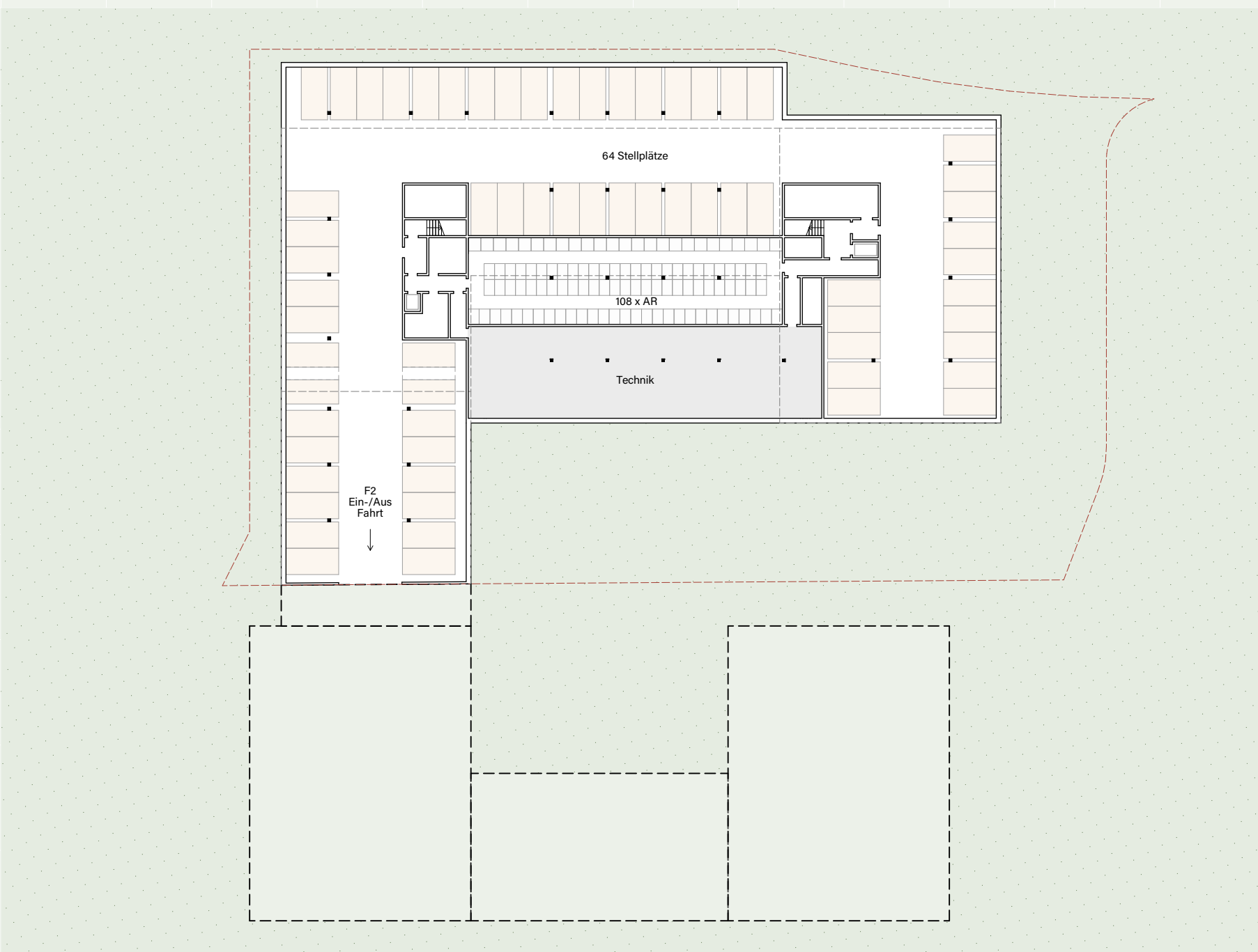
GRUNDRISS UTERGESCHOSS 1:500
