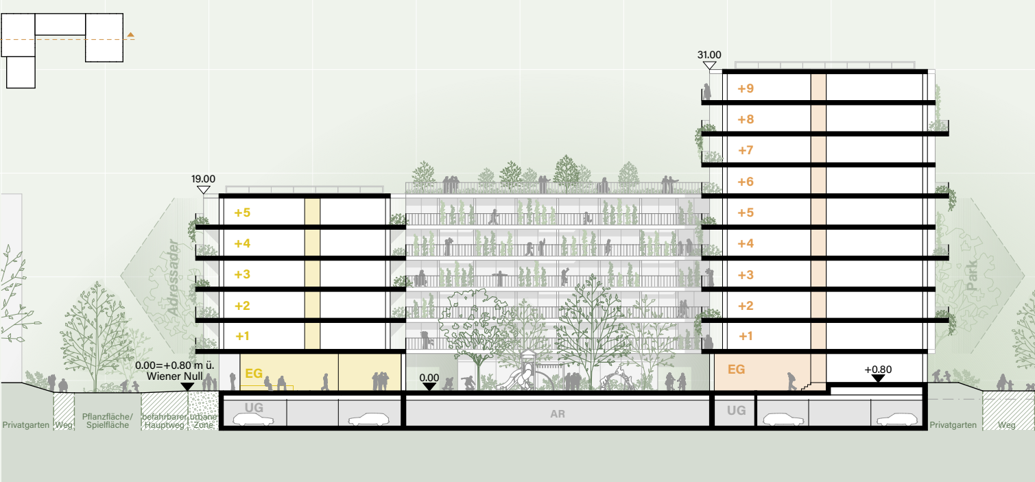
SCHNITT A 1:500
