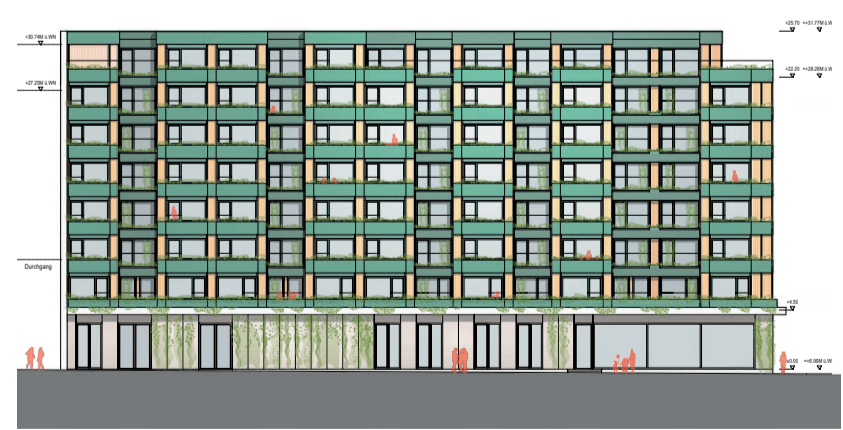
Ansicht Ost 1:200
